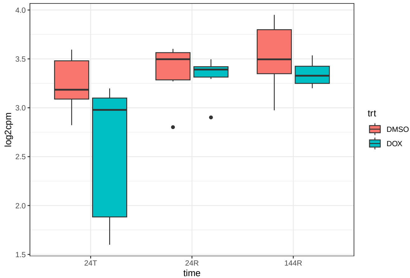
gene 148254 ZNF555
